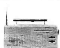
TR-803 S
